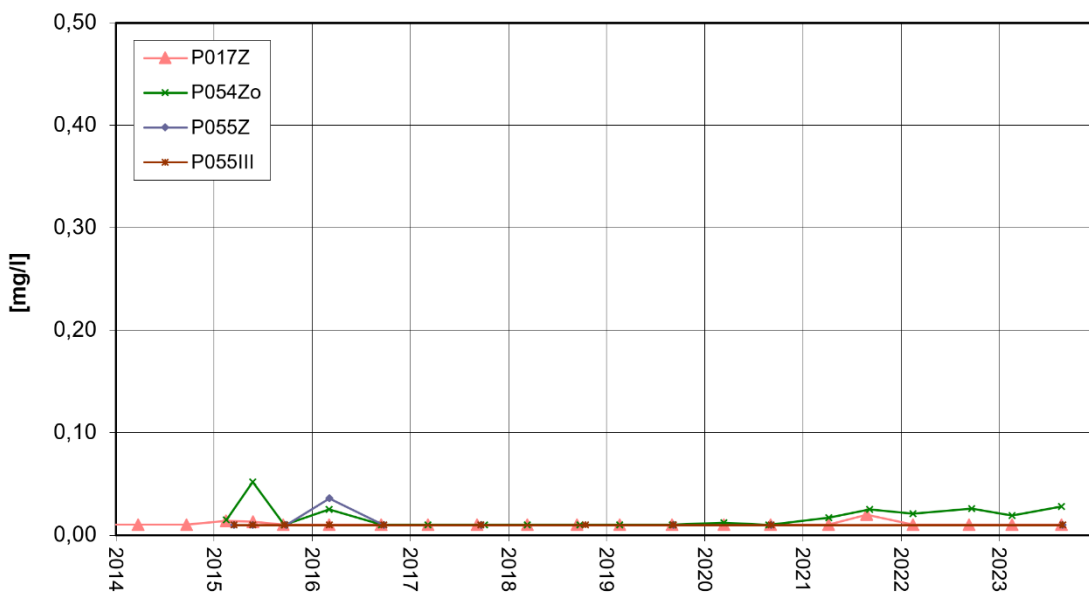
Nordrand Altabschnitte TBZ/TBIII AOX-Entwicklung
