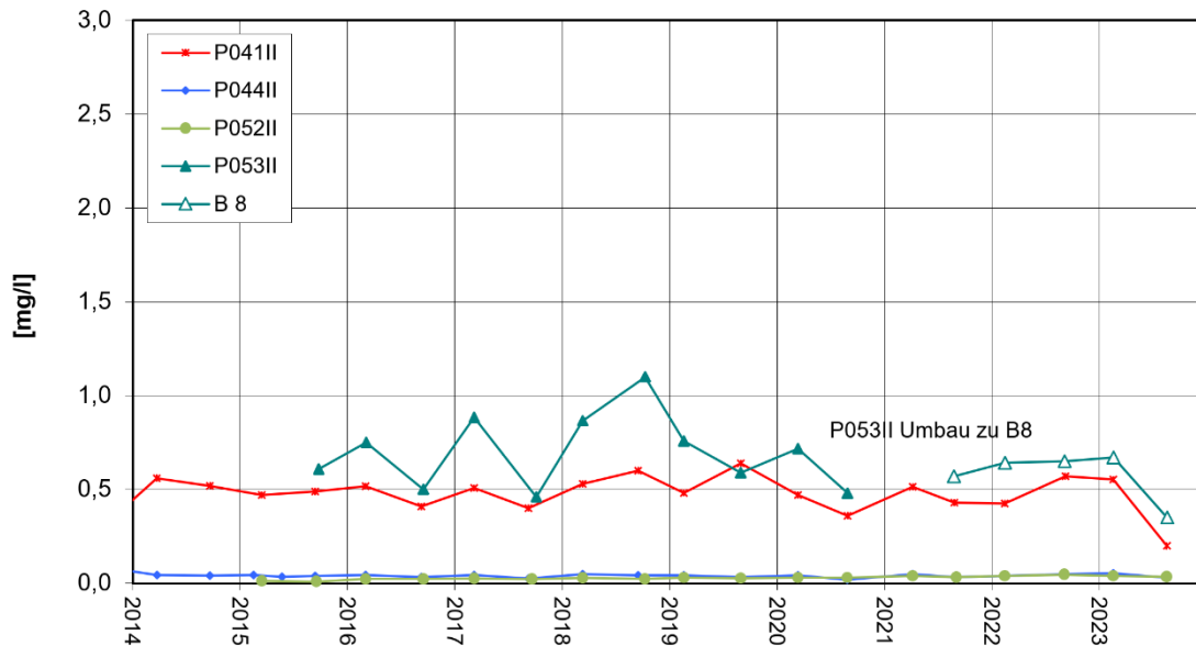
Nordwestrand Altabschnitte TBII Mecoprop-Entwicklung
