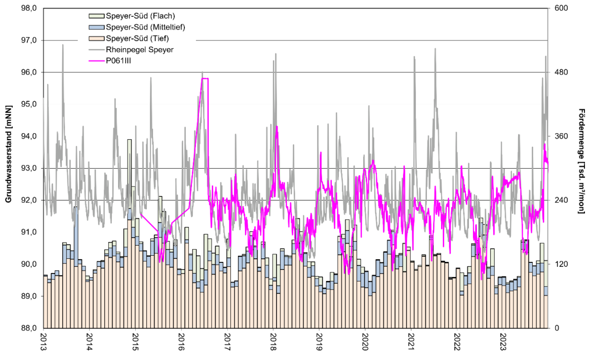
Entwicklung Grundwasserstände und Fördermenge Speyer-Süd sowie Rheinwasserstand Einfachesstelle P061 (Nördlich Altrheinsystem)
