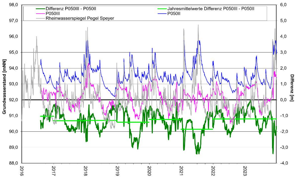
Entwicklung Grundwasserstände und Differenzen Tiefenbereiche III - II P050
