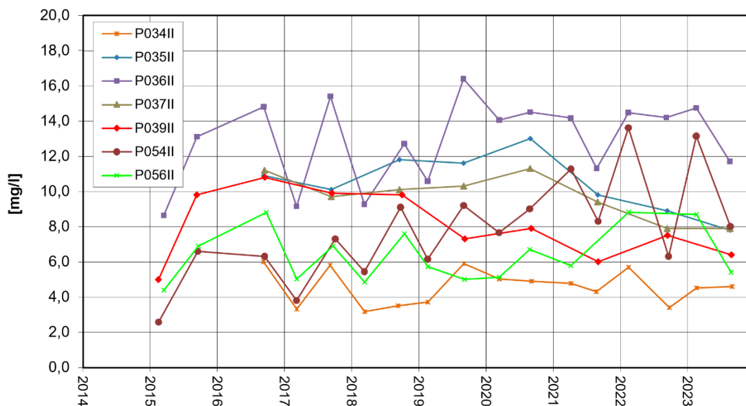
Nordrand Altabschnitte TBI Summe 1,4-Dioxan + 1,3,5-Trioxan-Entwicklung
