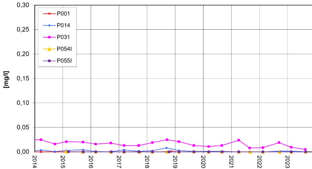
Nordrand Altabschnitte TBI Mecoprop-Entwicklung
