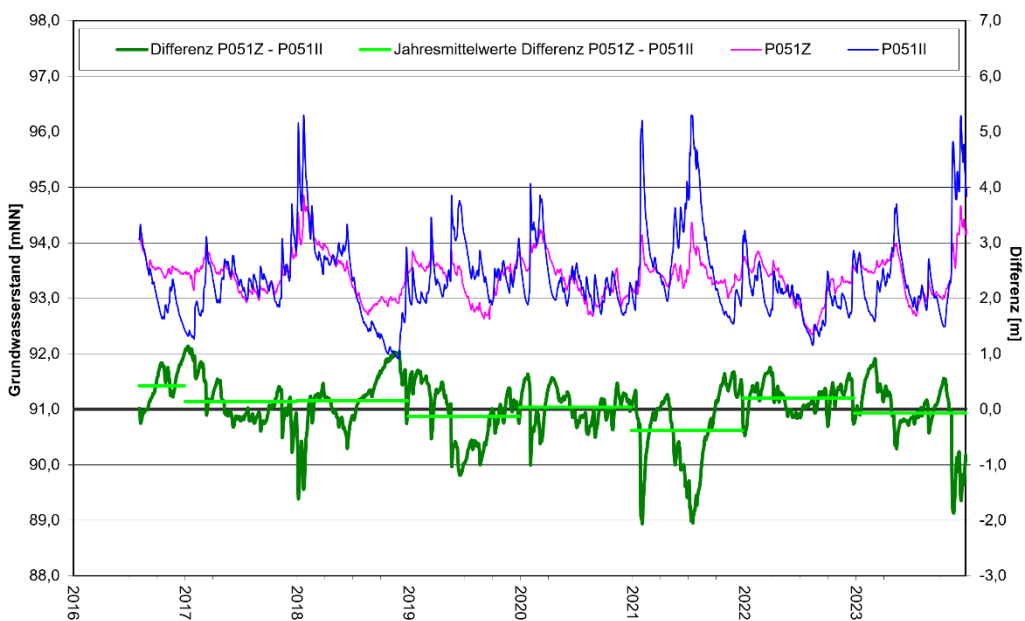
Entwicklung Grundwasserstände und Differenzen Tiefenbereiche Z - II P051
