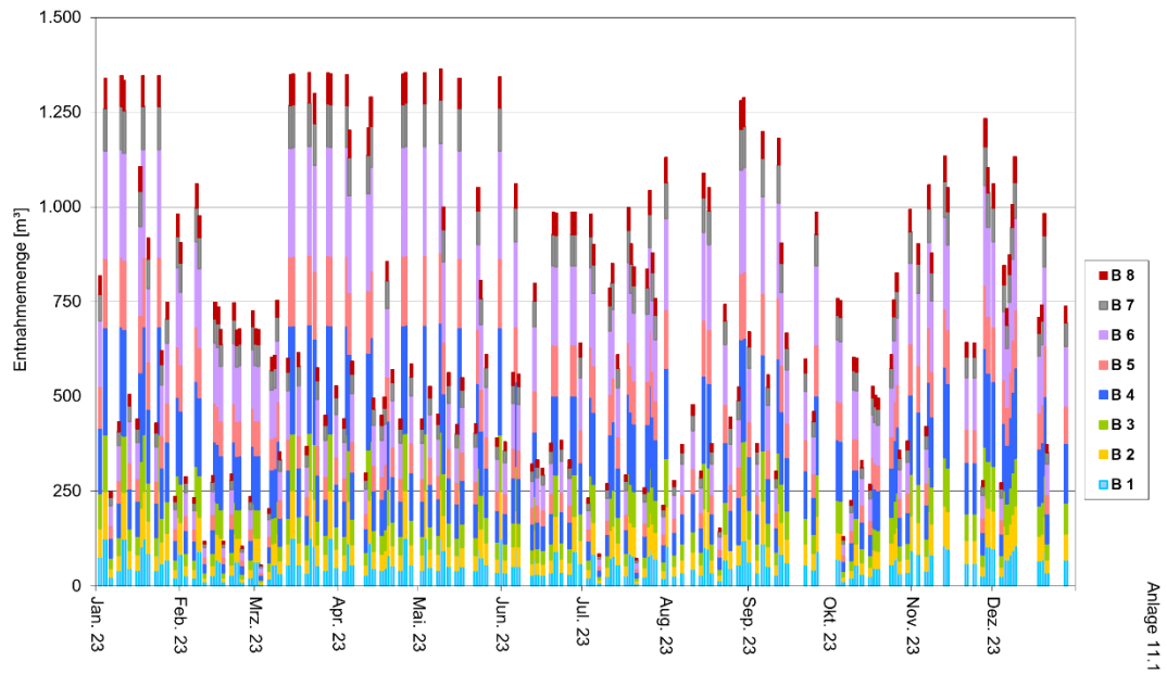
Fördermengen 2023 an den Sanierungsbrunnen B1 bis B8 Fördermengen der einzelnen Abpumpmaßnahmen
