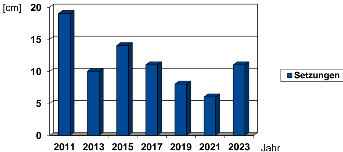
Diagramm 6: Entwicklung der Setzungen am Filterkuchenfeld II
