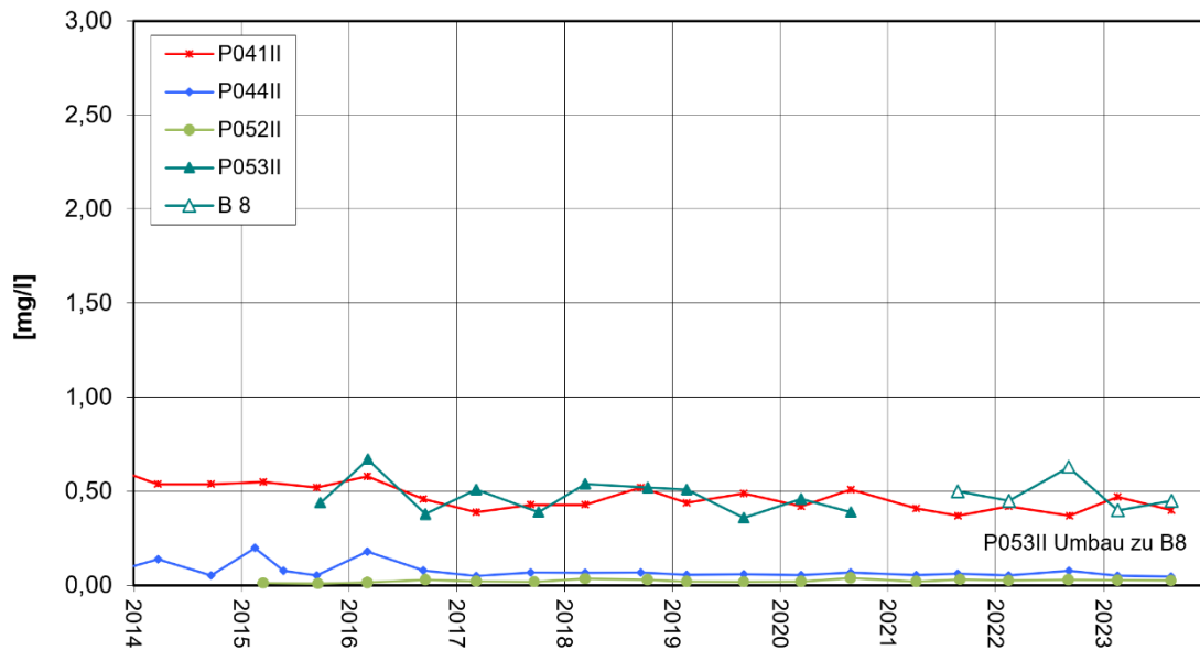
Nordwestrand Altabschnitte TBII AOX-Entwicklung
