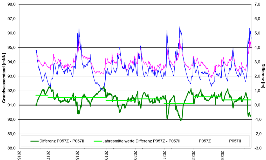
Entwicklung Grundwasserstände und Differenzen Tiefenbereiche Z - II P057
