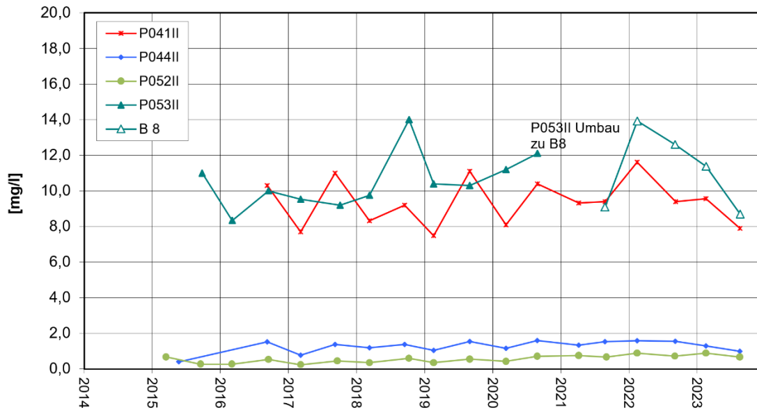
Nordwestrand Altabschnitte TBII Summe 1,4-Dioxan + 1,3,5-Trioxan-Entwicklung
