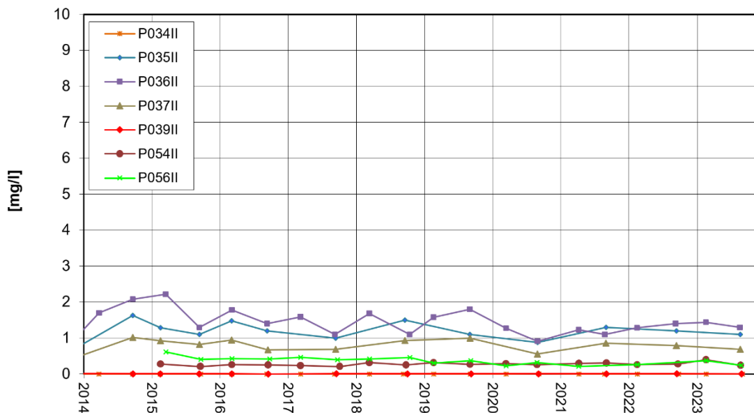
Nordrand Altabschnitte TBII Bentazon-Entwicklung
