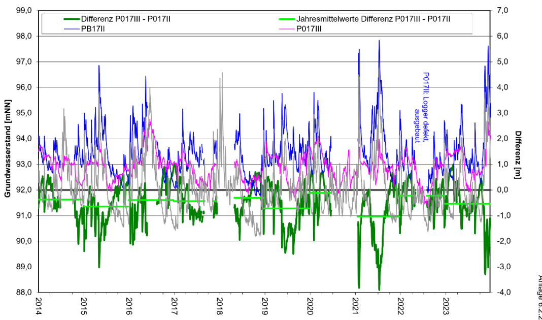
Entwicklung Grundwasserstände und Differenzen Tiefenbereiche III - II P017
