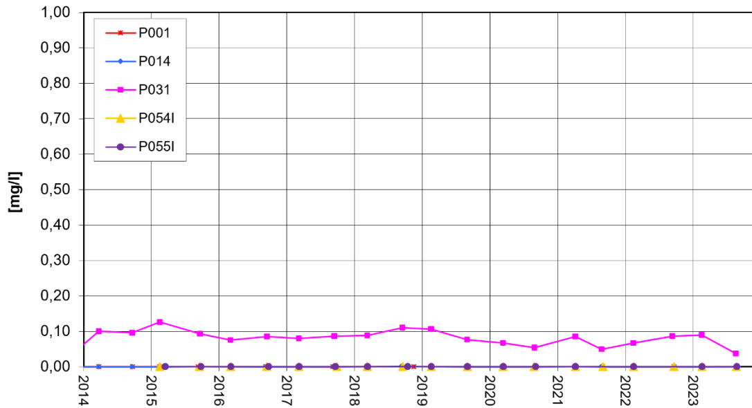
Nordrand Altabschnitte TBI Bentazon-Entwicklung
