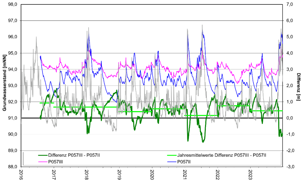
Entwicklung Grundwasserstände und Differenzen Tiefenbereiche III - II P057
