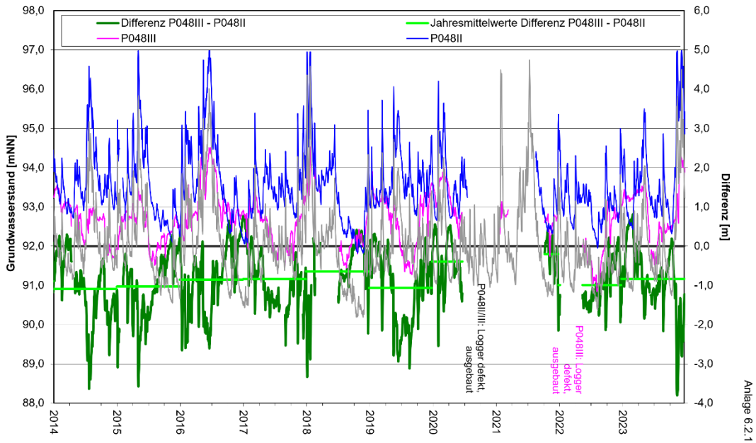
Entwicklung Grundwasserstände und Differenzen Tiefenbereiche III - II P048
