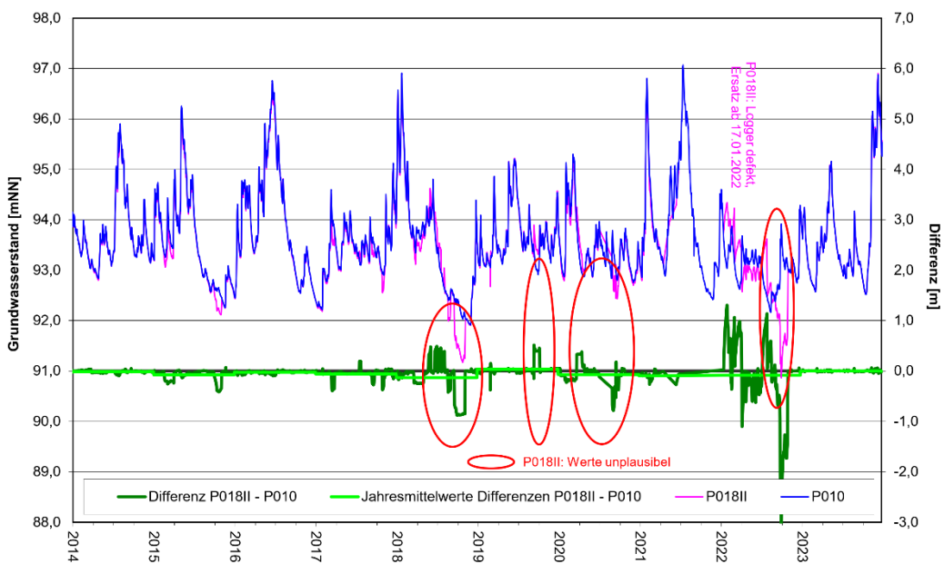
Entwicklung Grundwasserstände und Differenzen Tiefenbereiche II - I P018II / P010
