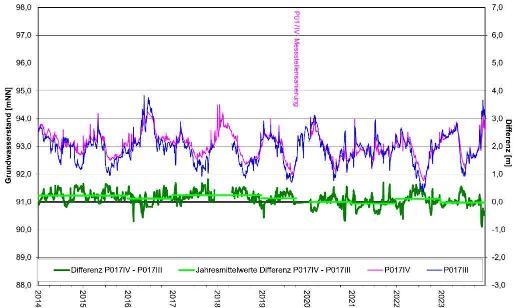
Entwicklung Grundwasserstände und Differenzen Tiefenbereiche IV - III P017
