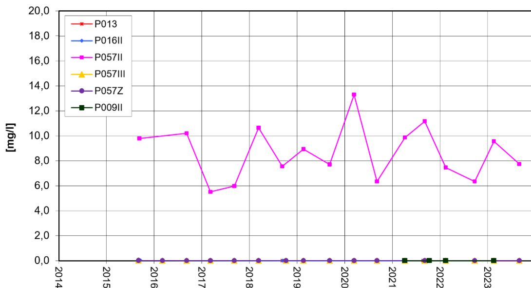
Anstrom Deponie Summe Sulfonsäuren-Entwicklung
