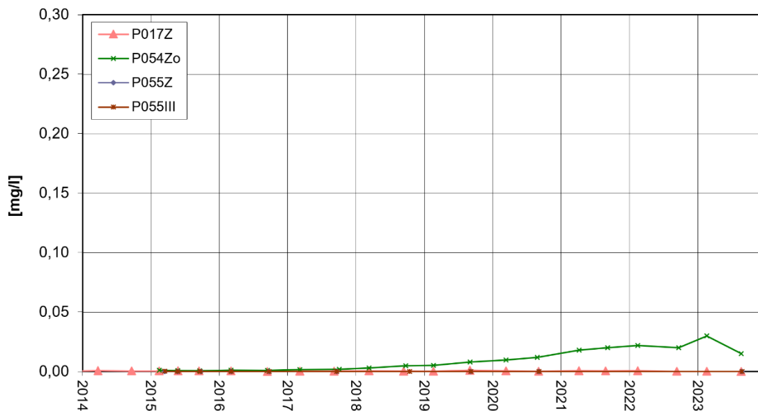
Nordrand Altabschnitte TBZ/TBIII Mecoprop-Entwicklung
