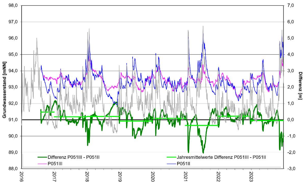
Entwicklung Grundwasserstände und Differenzen Tiefenbereiche III - II P051
