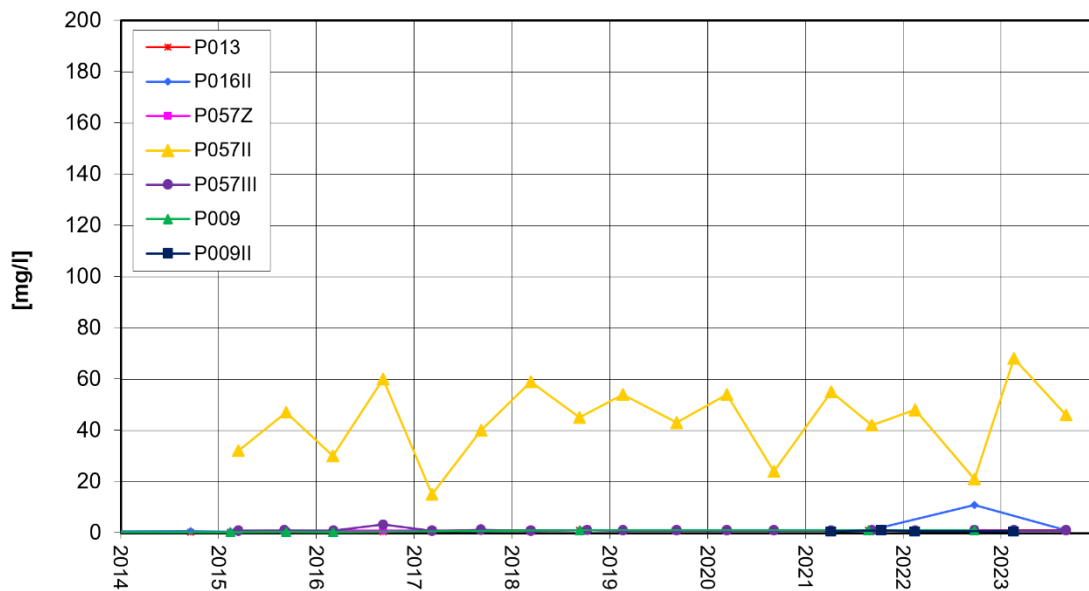
Anstrom Deponie Ammonium-Entwicklung
