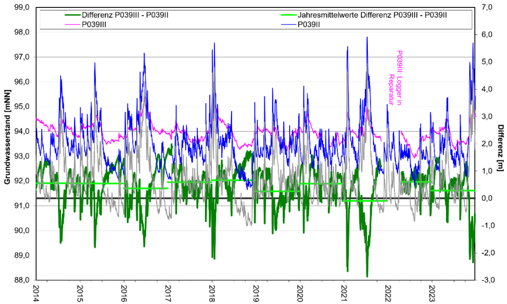
Entwicklung Grundwasserstände und Differenzen Tiefenbereiche III - II P039
