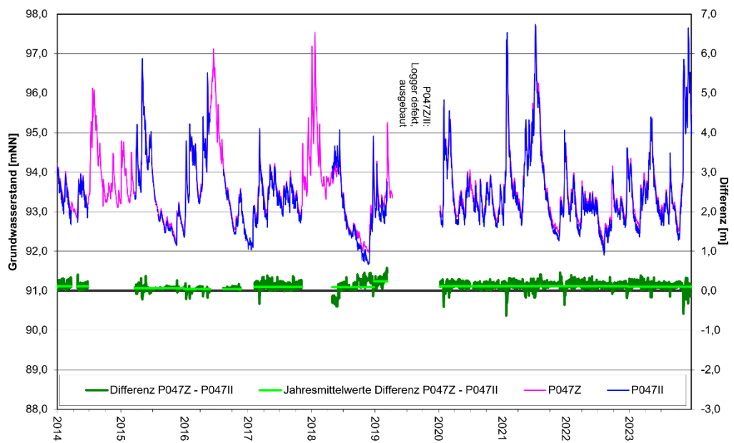
Entwicklung Grundwasserstände und Differenzen Tiefenbereiche Z - II P047
