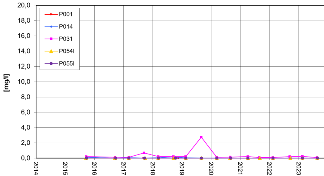
Nordrand Altabschnitte TBI Summe Sulfonsäuren-Entwicklung
