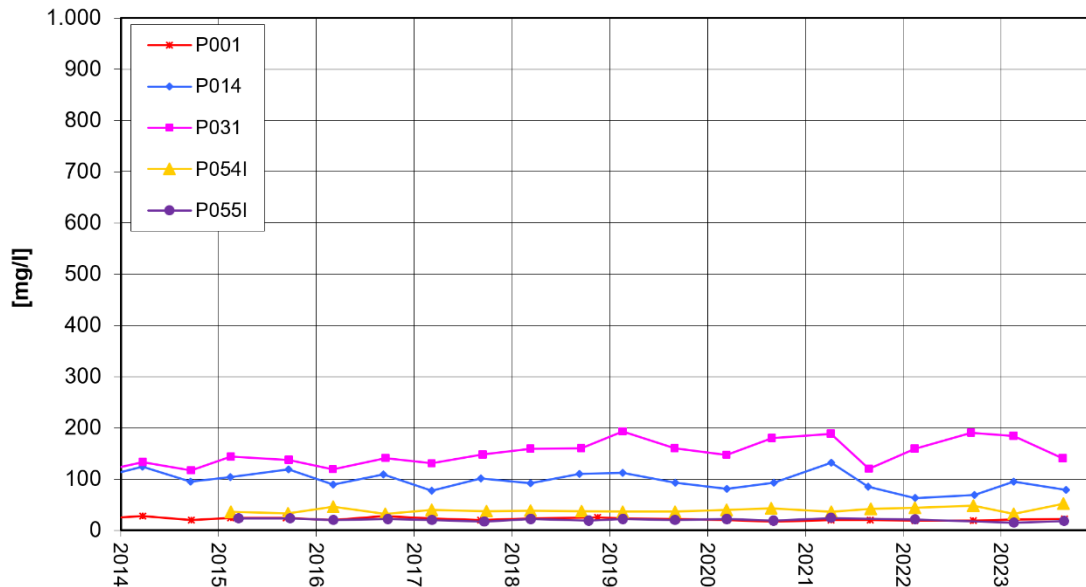
Nordrand Altabschnitte TBI Chlorid-Entwicklung
