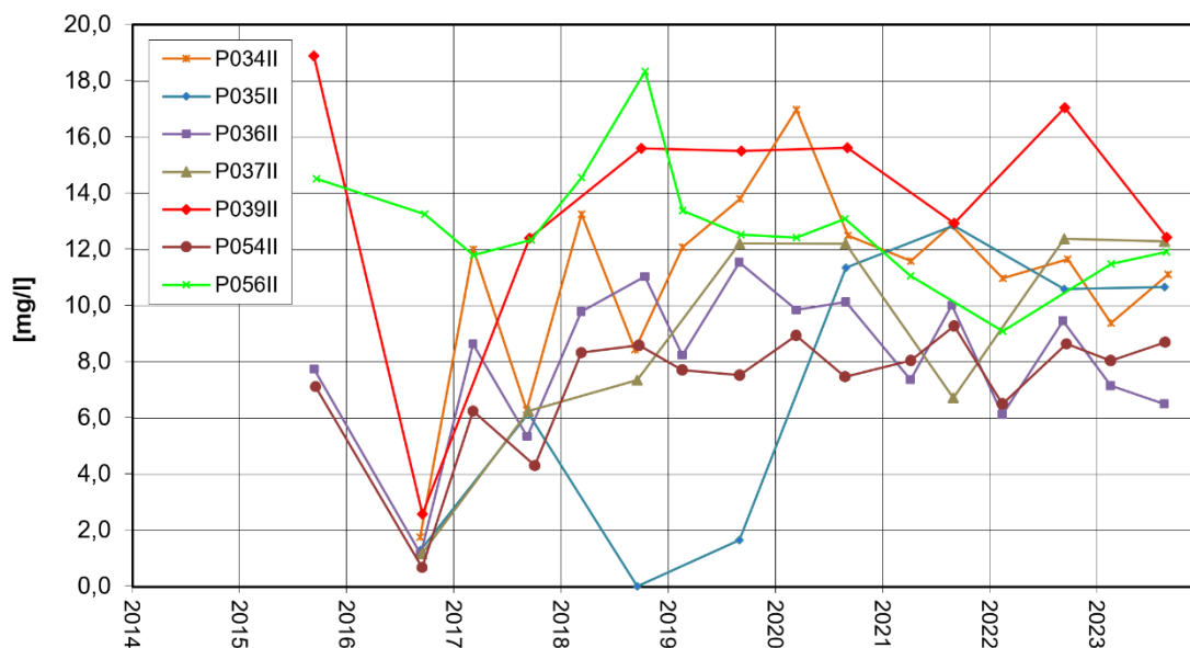
Nordrand Altabschnitte TBII Summe Sulfonsäuren-Entwicklung
