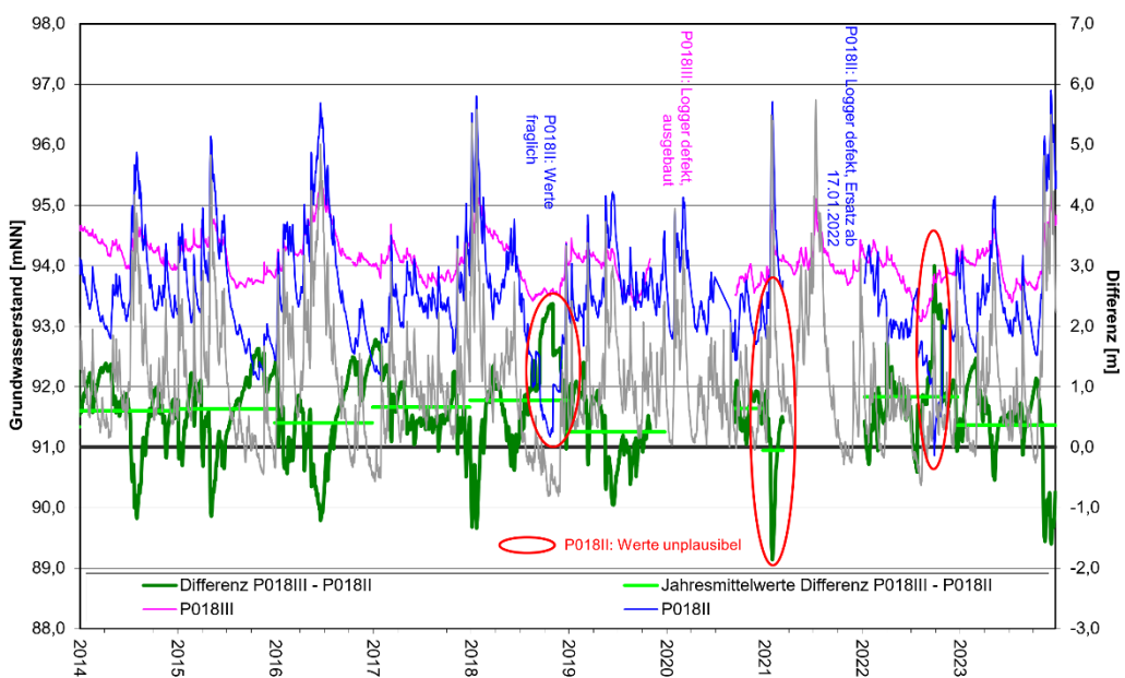
Entwicklung Grundwasserstände und Differenzen Tiefenbereiche III - II P018
