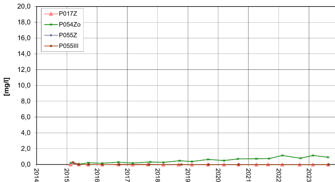
Nordrand Altabschnitte TBZ/TBIII Summe 1,4-Dioxan + 1,3,5-Trioxan-Entwicklung
