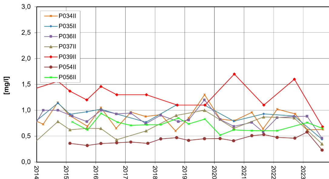
Nordrand Altabschnitte TBII Mecoprop-Entwicklung
