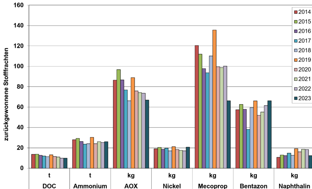
Abbildung 7: Stoffrückgewinnung an den Sanierungsbrunnen B1 bis B8 in den Betriebsjahren 2014 bis 2023
