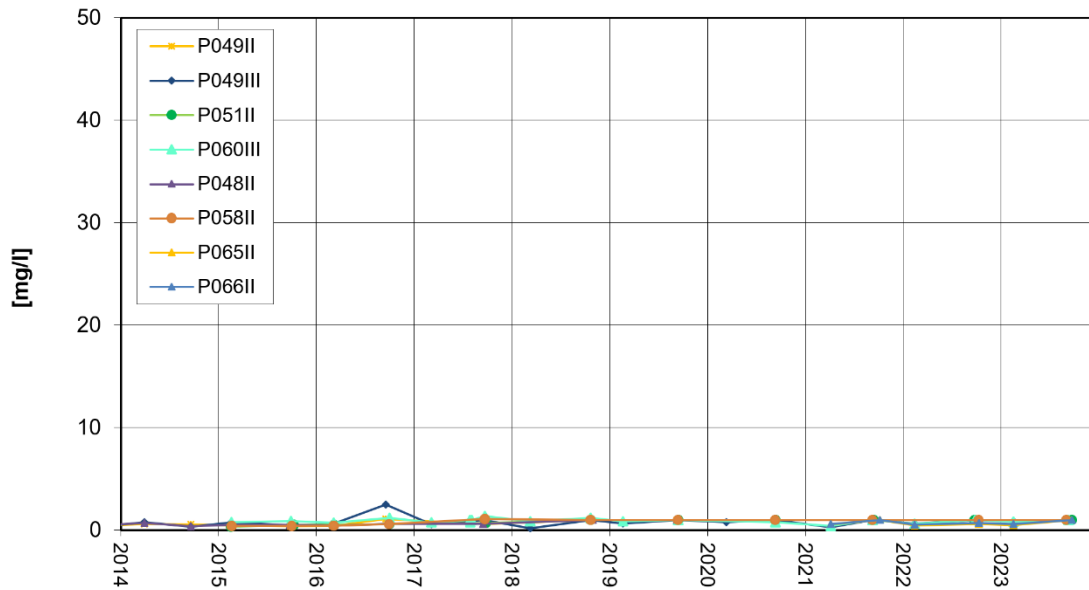
Nördlich Altrheinkanal Ammonium-Entwicklung
