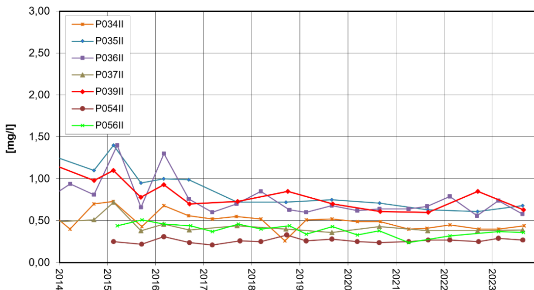
Nordrand Altabschnitte TBII AOX-Entwicklung
