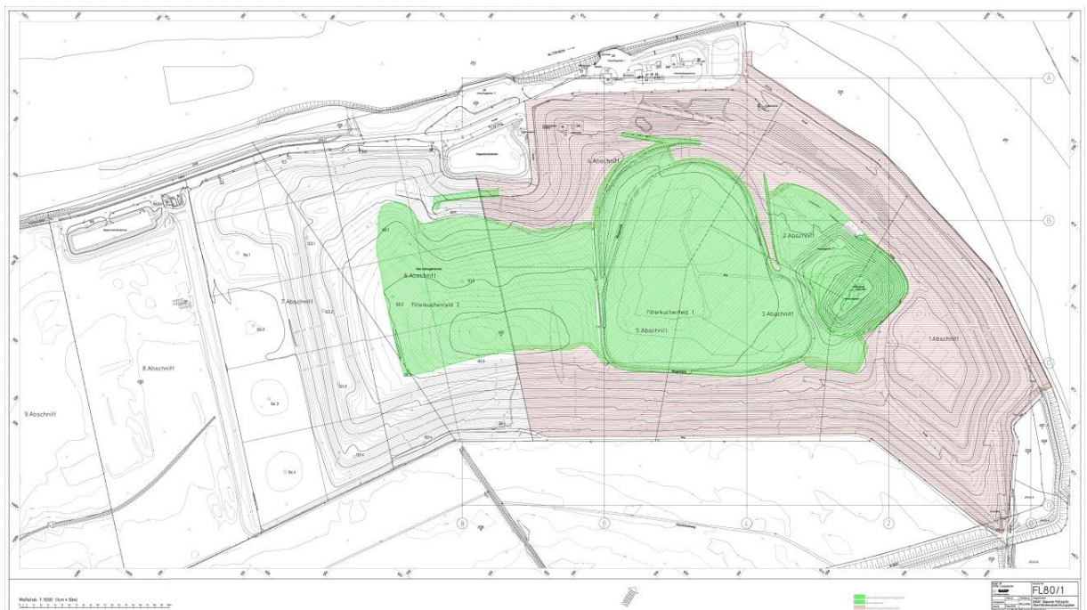
Lageplan 1: Oberflächenabdichtungssysteme Deponie Flotzgrün braun: Wasserhaushaltsschicht grün: Folienabdichtung
