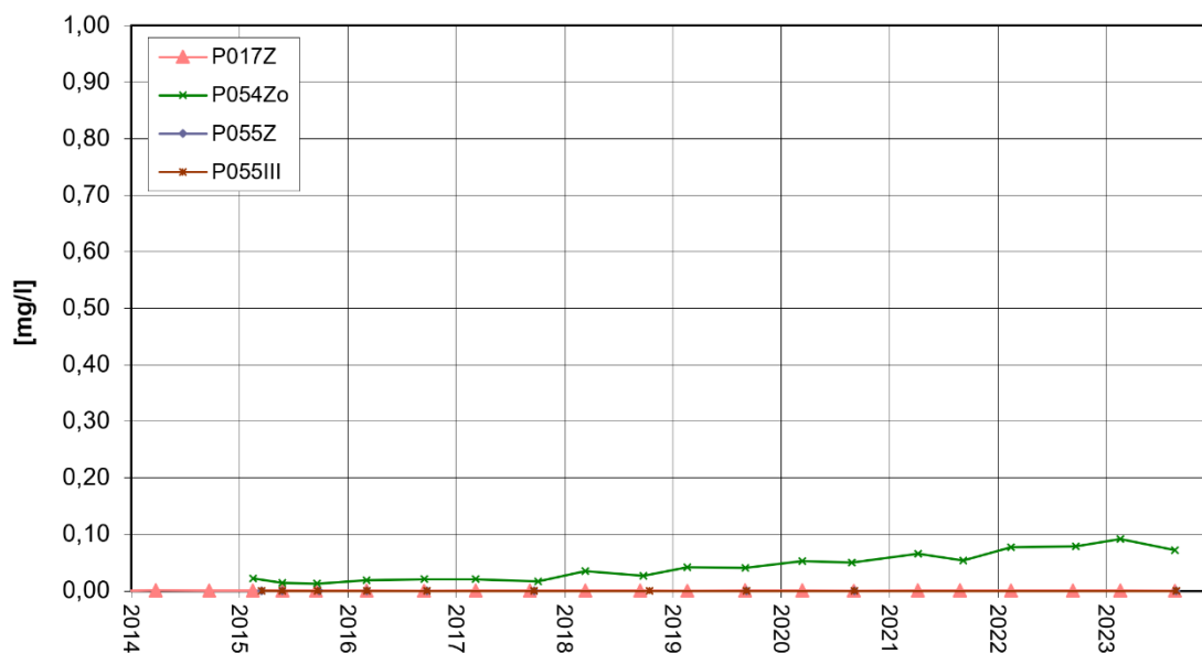
Nordrand Altabschnitte TBZ/TBIII Bentazon-Entwicklung
