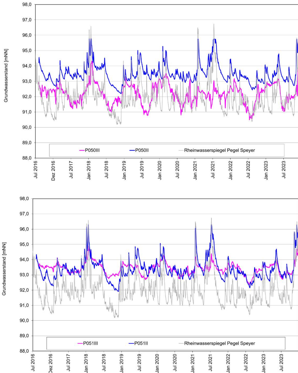
Abbildung 1: Entwicklung der Grundwasserstände an den Messstellen P050 (oben) und P051 (unten) in den TB II und III
