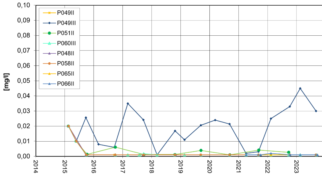
Nördlich Altrheinkanal Summe 1,4-Dioxan + 1,3,5-Trioxan-Entwicklung
