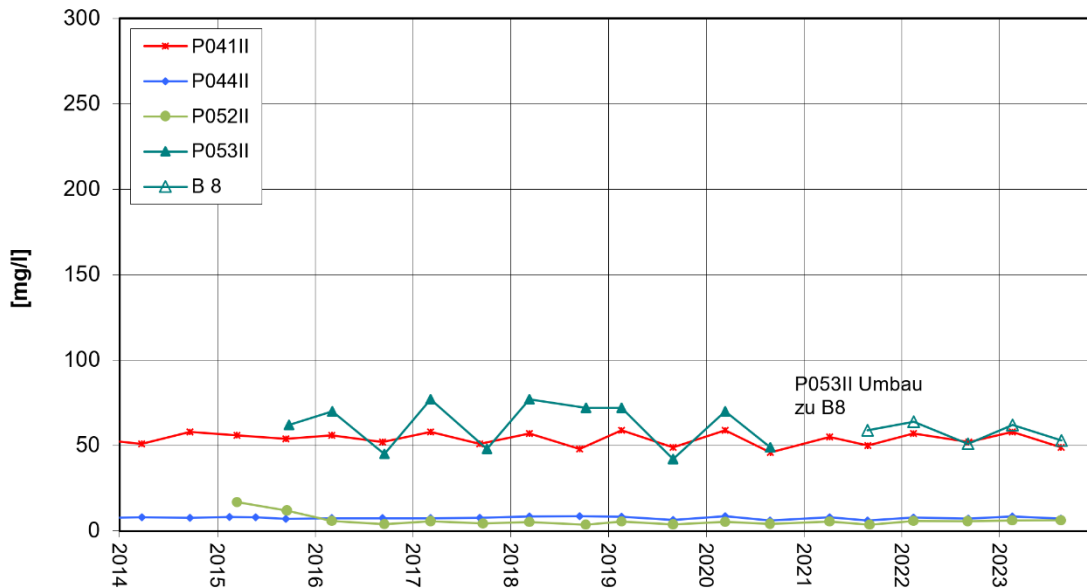
Nordwestrand Altabschnitte TBII DOC-Entwicklung
