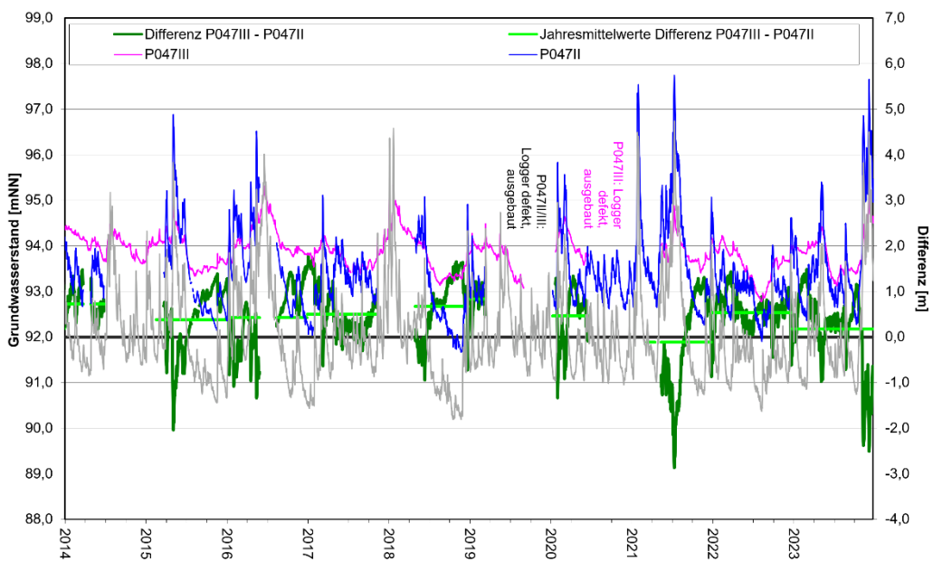
Entwicklung Grundwasserstände und Differenzen Tiefenbereiche III - II P047
