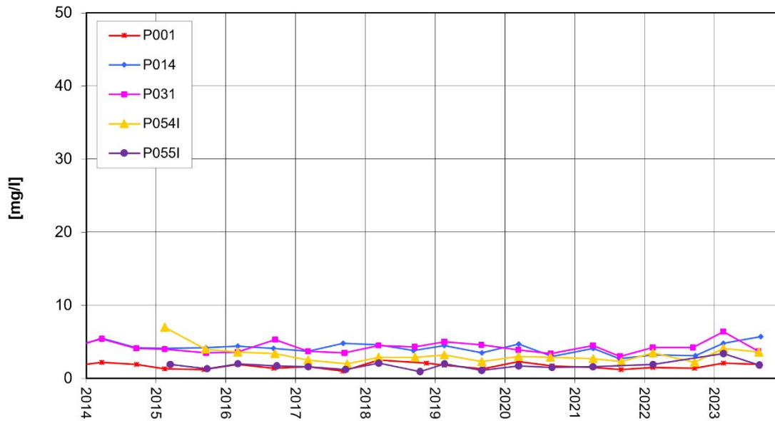
Nordrand Altabschnitte TBI DOC-Entwicklung
