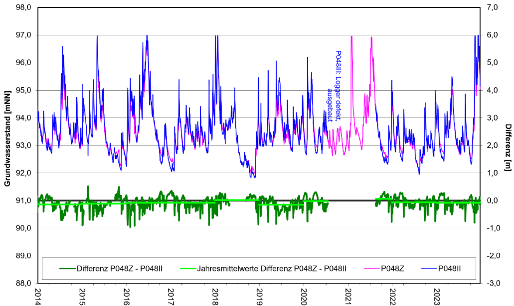
Entwicklung Grundwasserstände und Differenzen Tiefenbereiche Z - II P048
