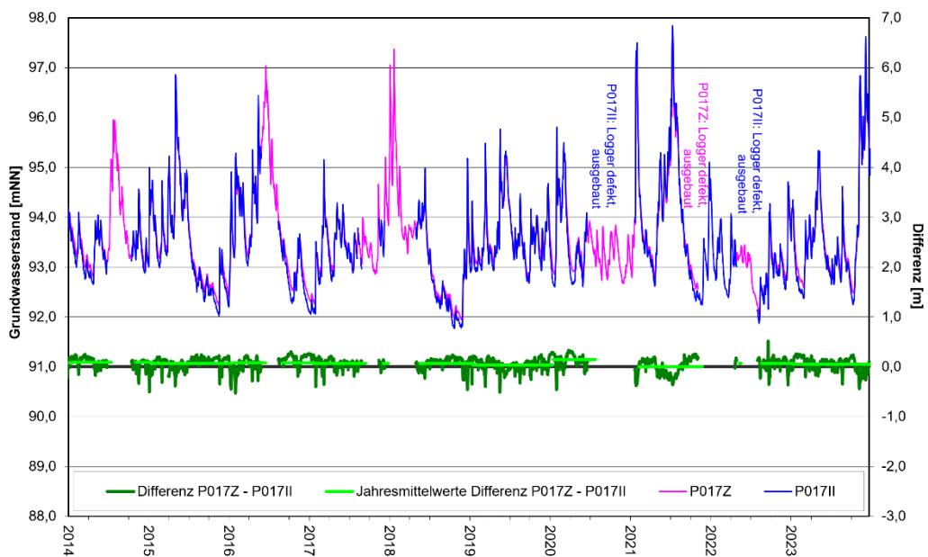
Entwicklung Grundwasserstände und Differenzen Tiefenbereiche Z - II P017
