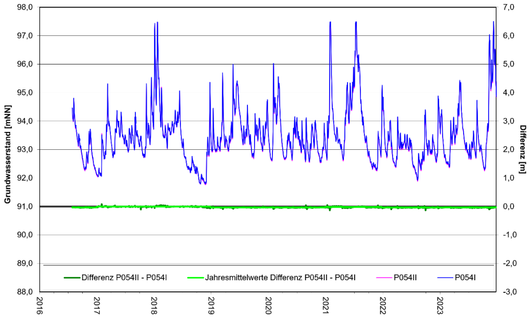
Entwicklung Grundwasserstände und Differenzen Tiefenbereiche II - I P054
