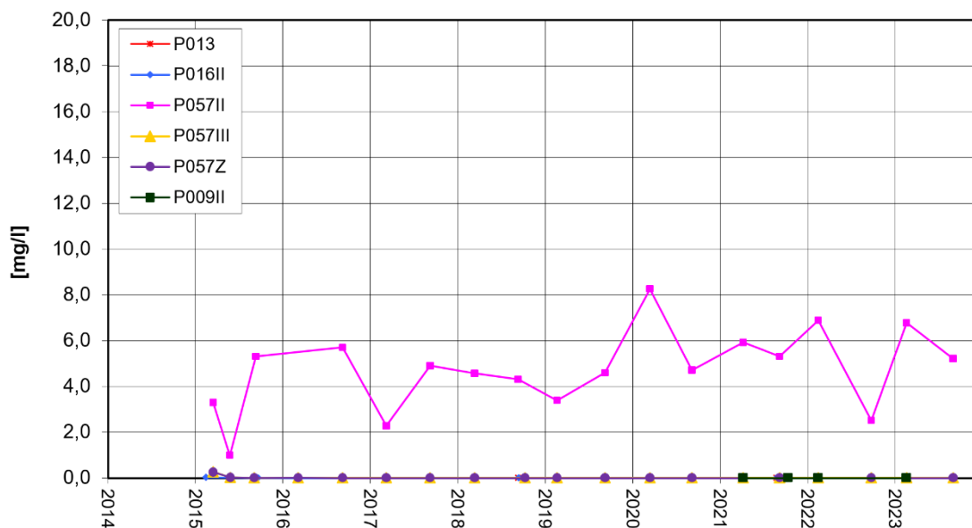
Anstrom Deponie Summe 1,4-Dioxan + 1,3,5-Trioxan-Entwicklung
