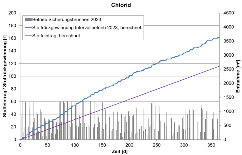
Abbildung 9: Entwicklung der berechneten Stoffströme 2023 für Chlorid
