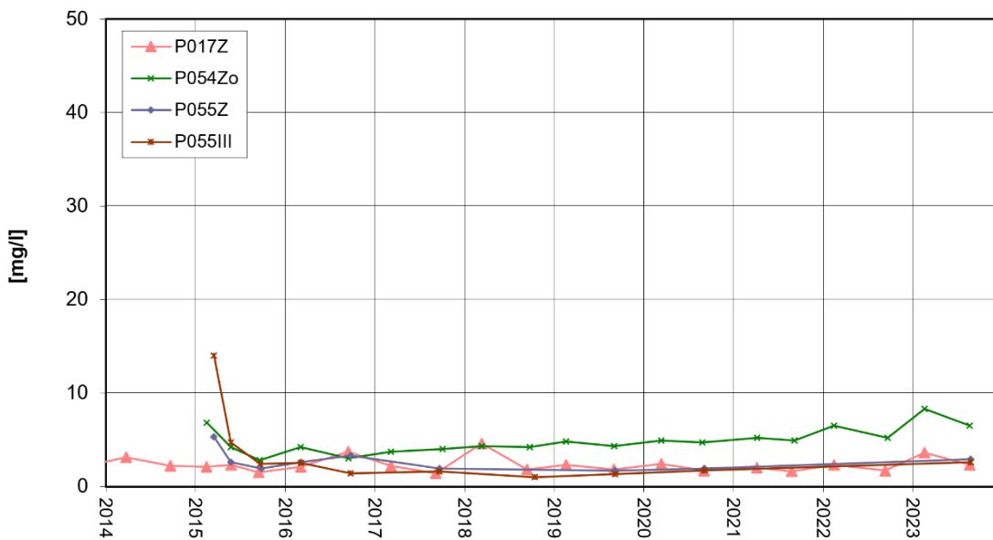
Nordrand Altabschnitte TBZ/TBIII DOC-Entwicklung
