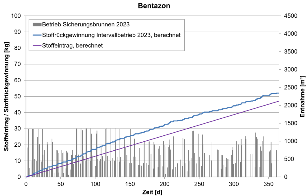
Abbildung 11: Entwicklung der berechneten Stoffströme 2023 für Bentazon
