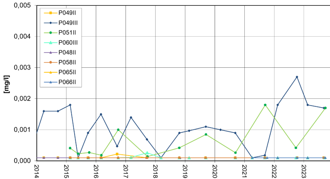
Nördlich Altrheinkanal Mecoprop-Entwicklung
