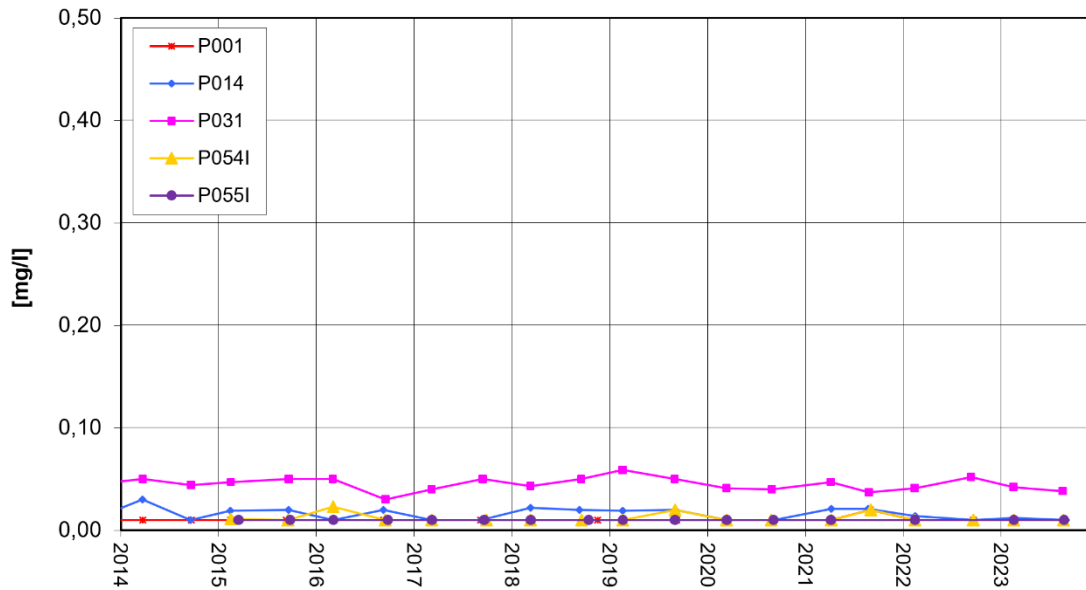
Nordrand Altabschnitte TBI AOX-Entwicklung
