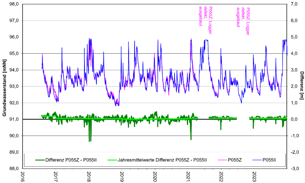
Entwicklung Grundwasserstände und Differenzen Tiefenbereiche Z - II P055
