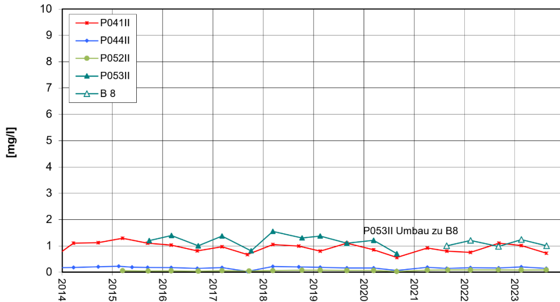
Nordwestrand Altabschnitte TBII Bentazon-Entwicklung
