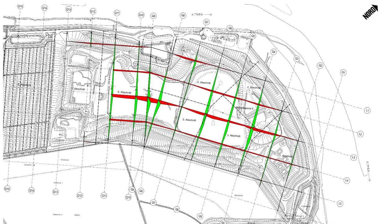
Lageplan 2: Ergebnis der Setzungsmessungen 2023
