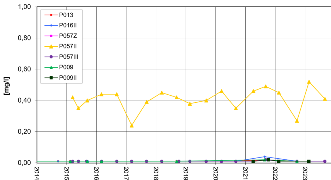
Anstrom Deponie AOX-Entwicklung
