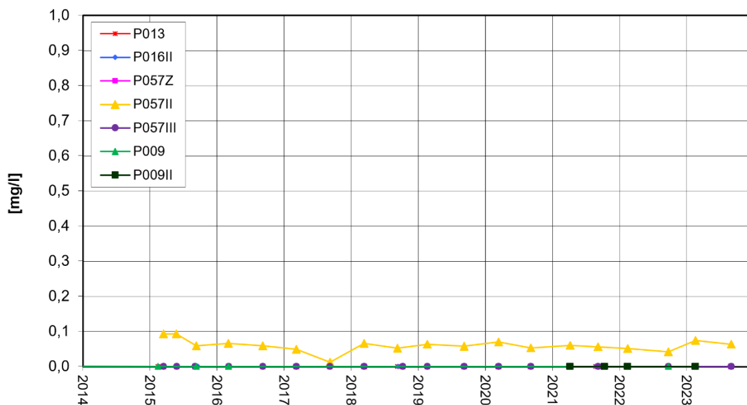
Anstrom Deponie Bentazon-Entwicklung
