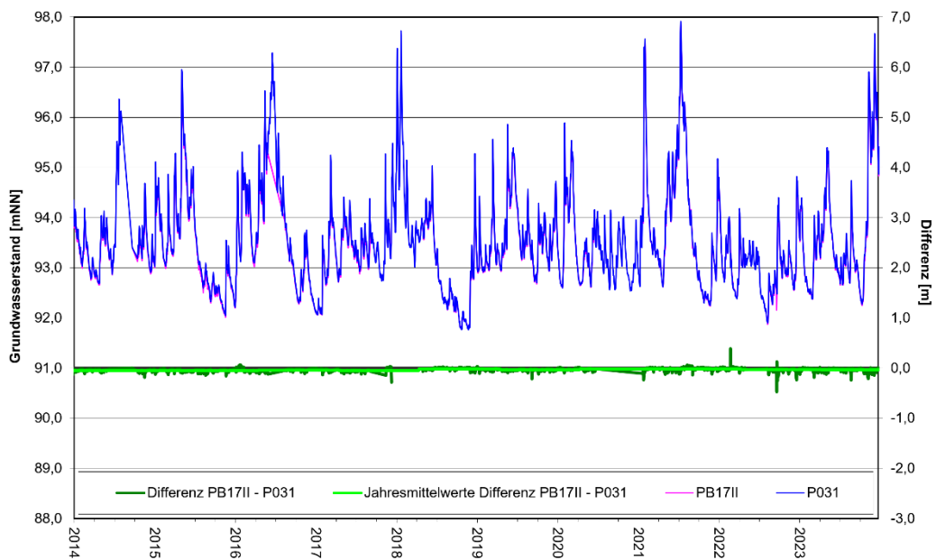
Entwicklung Grundwasserstände und Differenzen Tiefenbereiche II - I PB17II / P031
