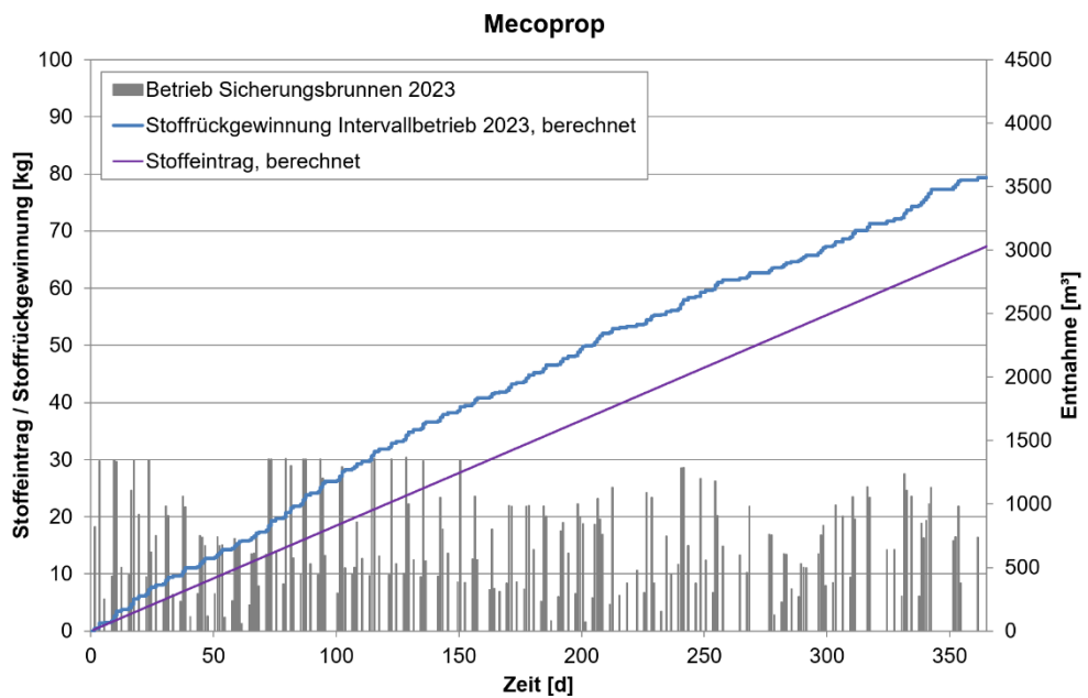
Abbildung 10: Entwicklung der berechneten Stoffströme 2023 für Mecoprop
